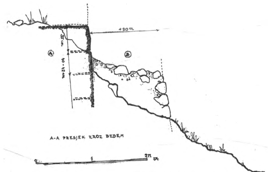
Sk. 5. — Presjek kroz ilirski odnosno ranoantički bedem na Gradini, uz dograđeno pojačanje bedema u vapnenoj žbuci, vjerojatno iz faze rimskog Rhisiniuma, u kasnoj antici. (A. Faber)
