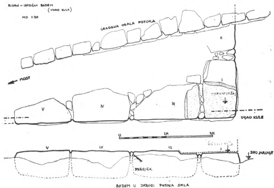
Sk. 6. — Tlocrt i presjek detalja u koritu rijeke Spile — donji bedemi na Carini (A. Faber)
