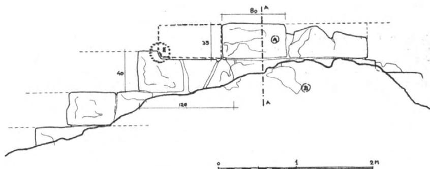
Sk. 4. — Detalj ilirskog, odnosno ranoantičkog bedema na Gradini (A. Faber)
